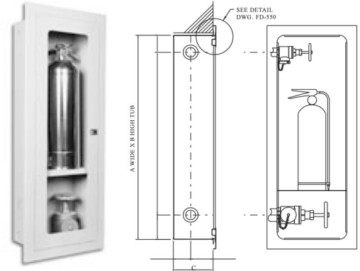
Model C-975E
