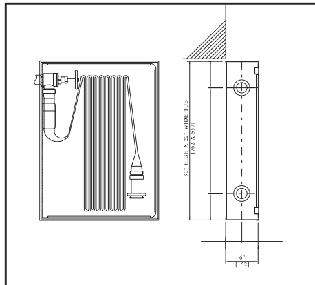
CS-400 (Single Valve)
