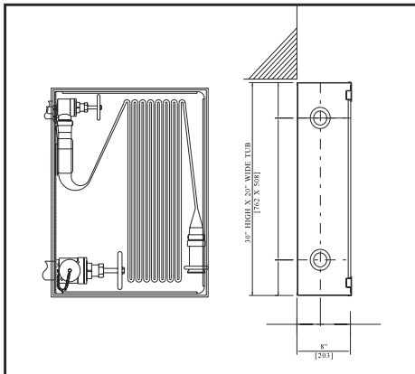
CS-200 (Double Valve)
